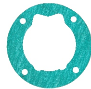
80.101.0022 JUNTA SUPERIOR DO CILÍNDRO TKJ-10NH TKJ-10SLC
