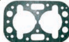
25.050.1064 JUNTA PLACA DE VÁLVULAS SUÇÃO FK5
