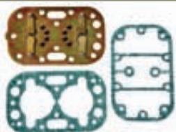
47.050.4754 CONJ. PLACA DE VÁLVULAS FK5 MODERNO
