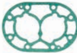
25.100.2122 JUNTA DA PLACA DE SUÇÃO 2N.2 / 4N.2 - 60 mm.
